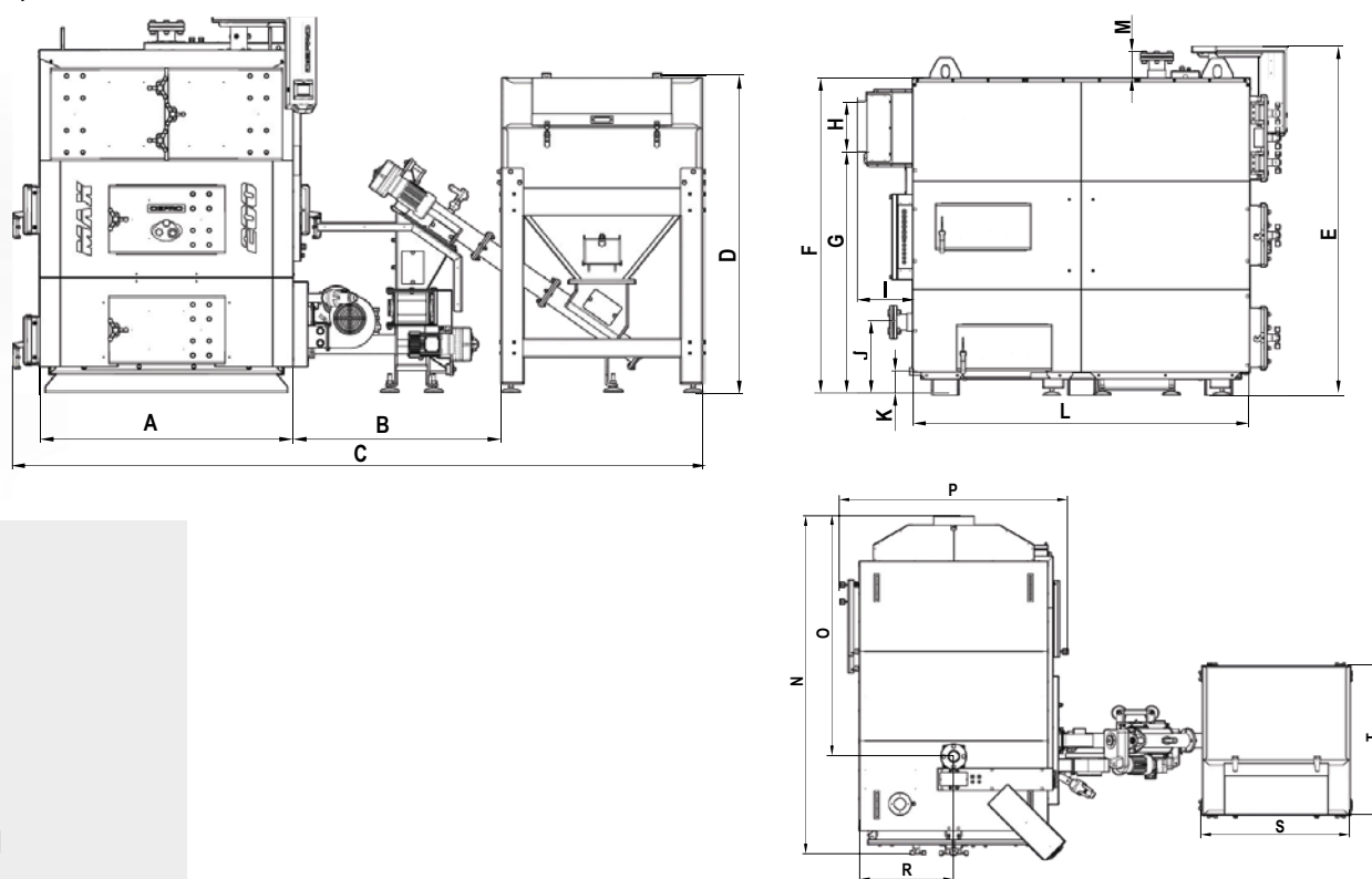
Wymiary kotła w mm
