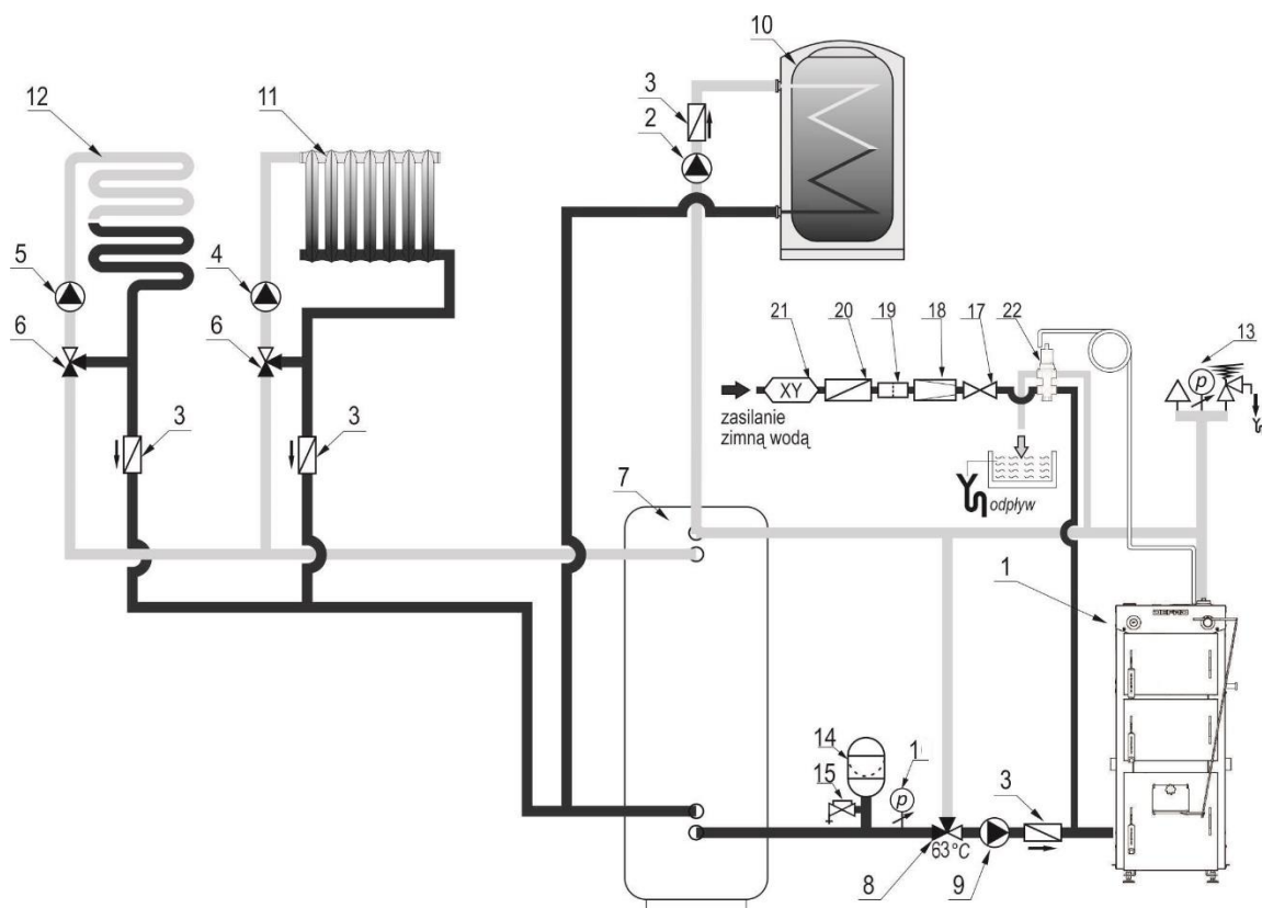
Rysunek 9. Uproszczony schemat instalacji grzewczej systemu zamkniętego.
