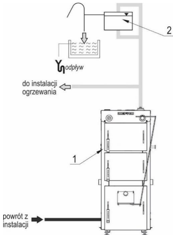
Rysunek 6. Przykładowy schemat zabezpieczeń kotła FIREWOOD:
