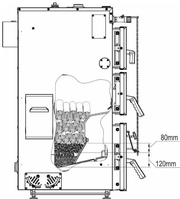
Rysunek 16. Prawidłowe ułożenie paliwa w komorze paleniskowej.
