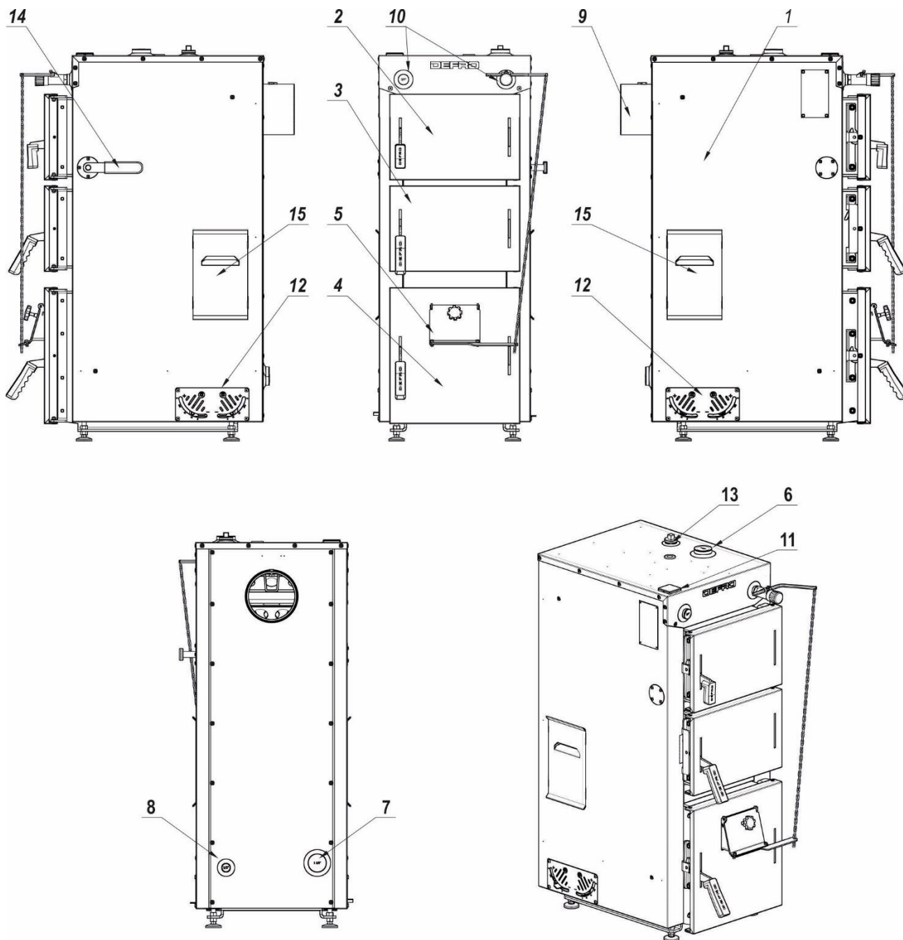
Rysunek 3. Podstawowe elementy kotła FIREWOOD
