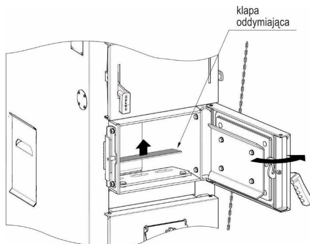
Rysunek 18. Klapa oddymiająca w przegrodzie paleniskowej.
