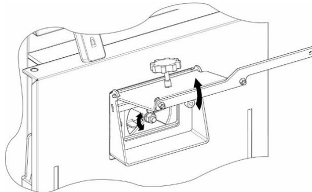
Rysunek 17. Przepustnica regulacji przepływu powietrza.
