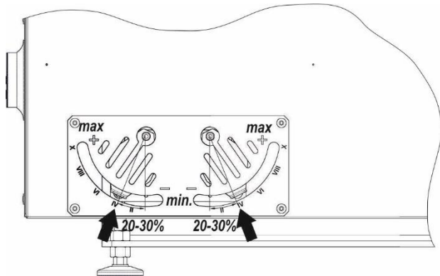
Rysunek 15. Ustawienie przepustnic powietrza wtórnego podczas rozpalania w kotle.
