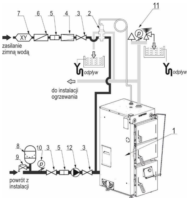
Rysunek 7. Przykładowy schemat zabezpieczeń kotła w układzie zamkniętym:
