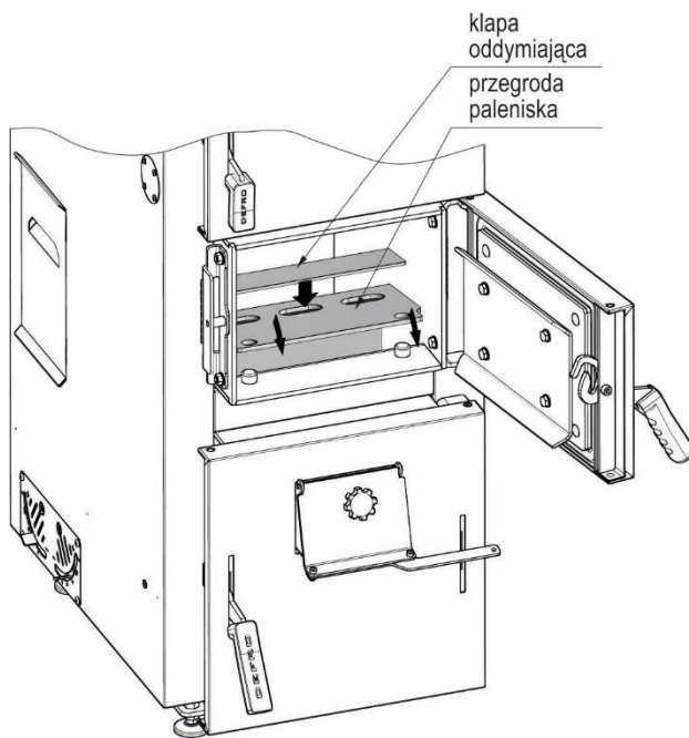
Rysunek 10. Montaż przegrody paleniska
