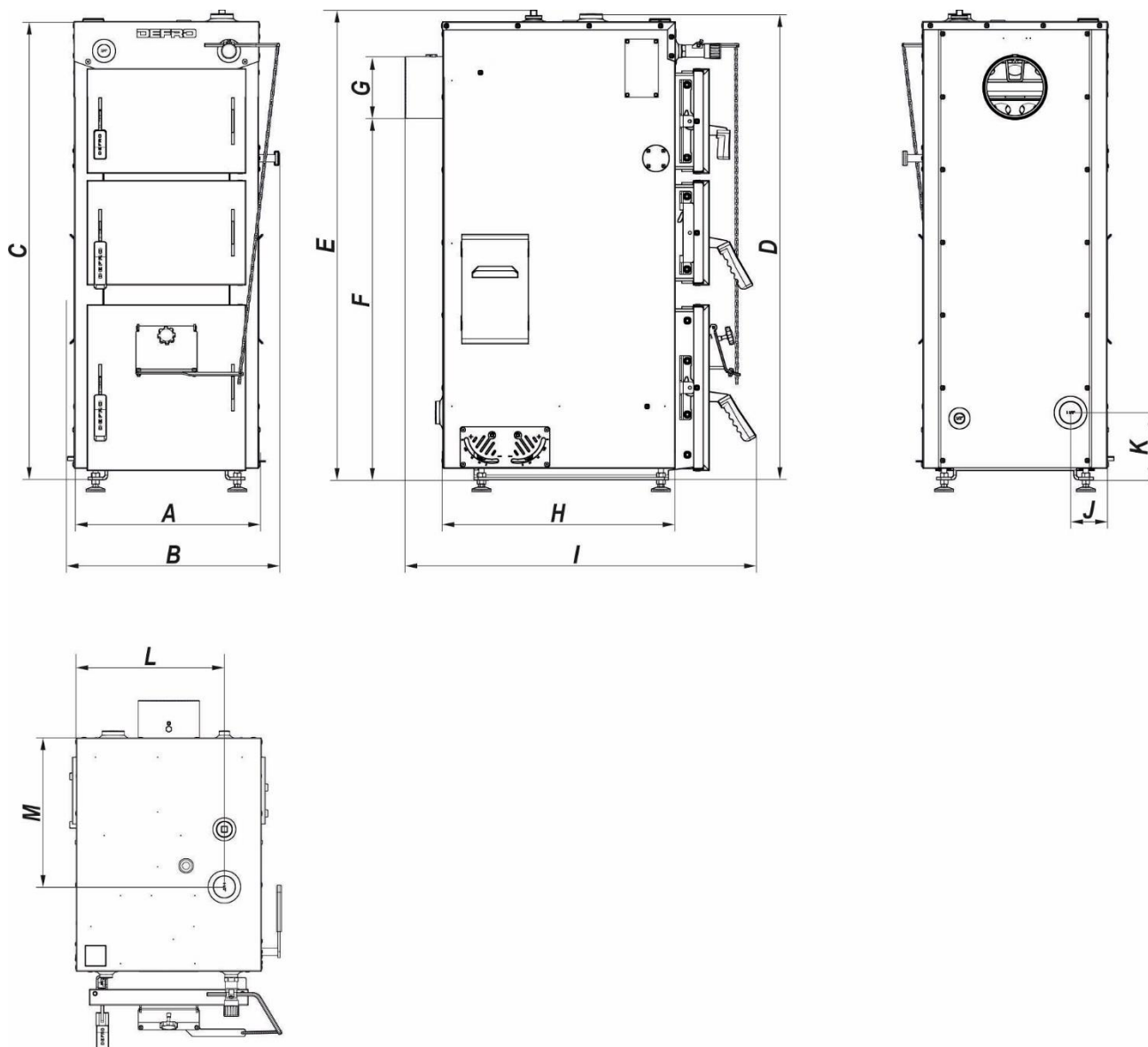
Rysunek 2. Podstawowe wymiary kotła FIREWOOD.
