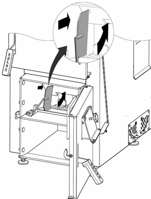
Rysunek 14. Przygotowanie przegrody paleniska do rozpalania.
